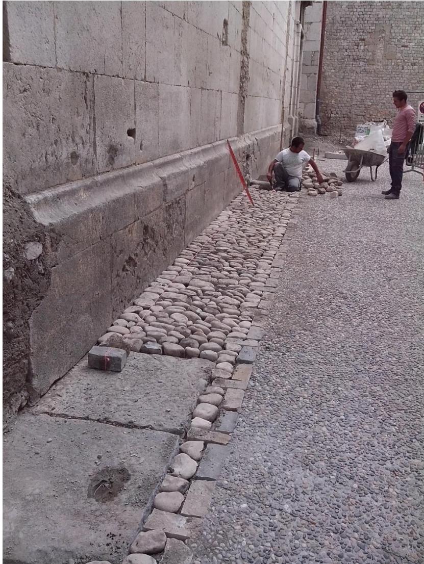
Construction de la calade sur. Au premier plan en bas à gauche, les dalles de fondation d'un contrefort aujourd'hui disparu, similaire à celui qu'on distingue en haut à gauche de l'image.
